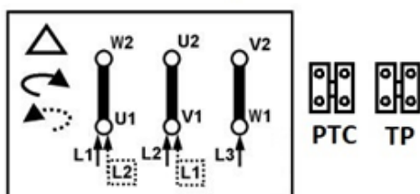
Dreieckschaltung
