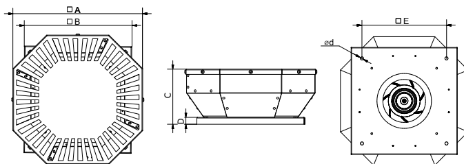
Rys. 2. Wymiary wentylatora VERT EC
