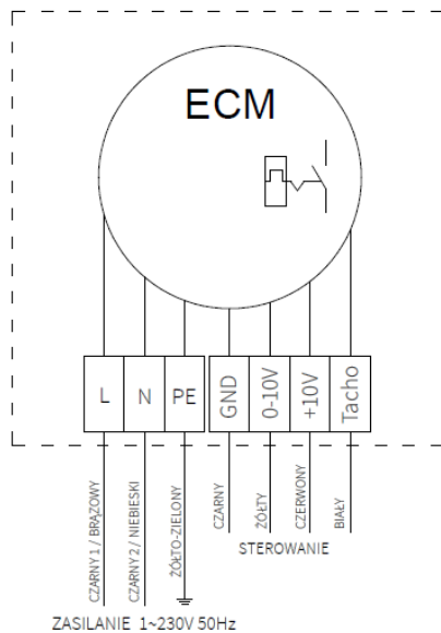
Rys. 3. Schemat połączeń
