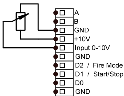
Przyłącze potencjometru
