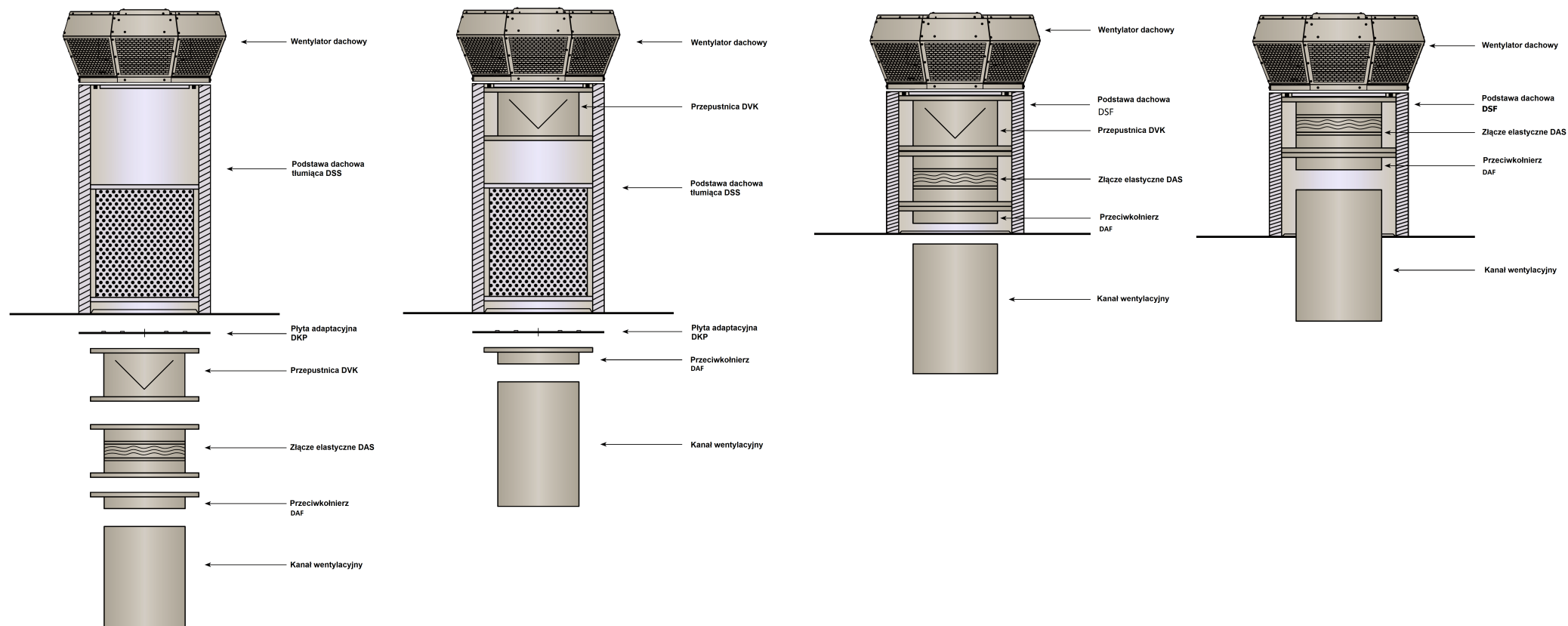
Przykład prawidłowego montażu wentylatorów dachowych na podstawach dachowych DSS i DSF
