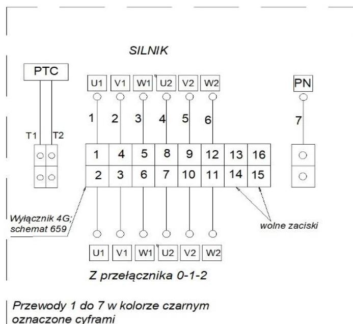
Schemat podłączenia dla silników dwubiegowych - wyłącznik serwisowy APATOR seria 4G
