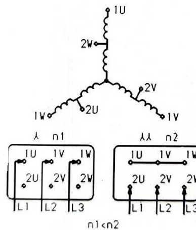
Schemat podłączenia silników dwubiegowych - puszka silnika
