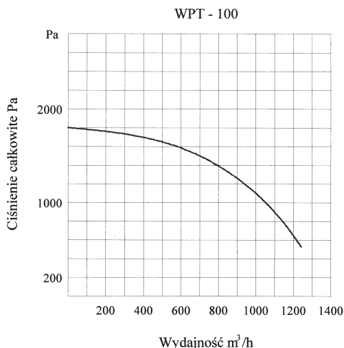
CHARAKTERYSTYKA PRACY WENTYLATORA WPT – 100
