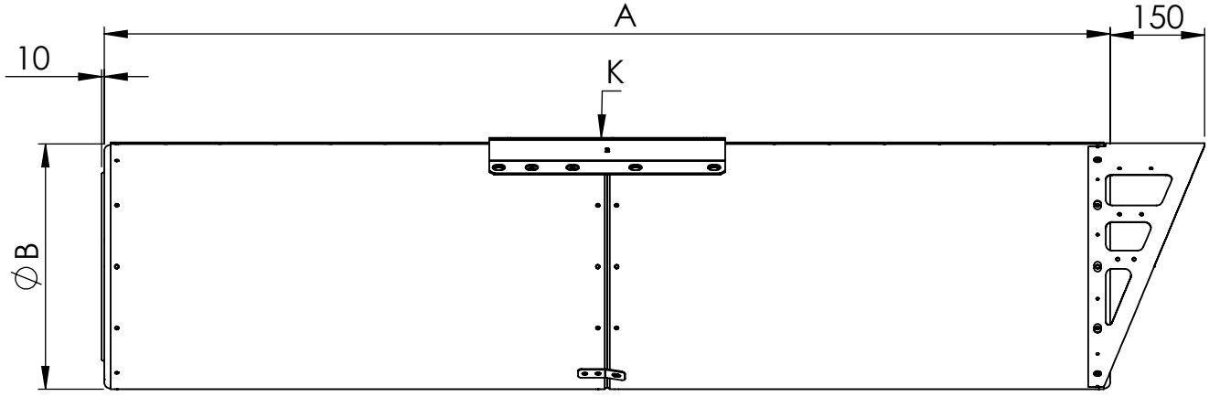
TEK YÖNLÜ JET FAN
