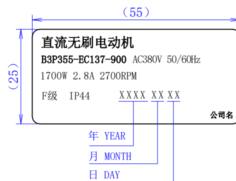
【铭牌一内容】
