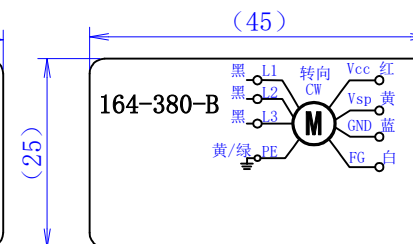
【铭牌二内容】
